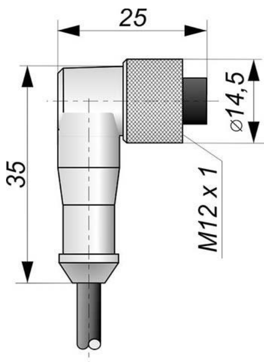
Габаритный чертеж
